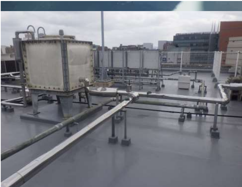
屋上
